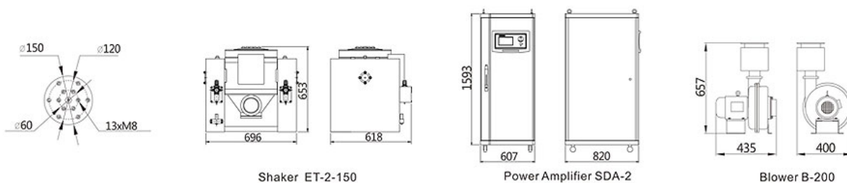
Shaker ET-2-150
