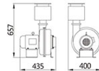
Blower B-200
