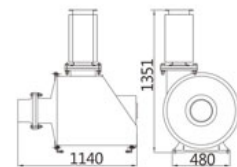
Blower B-2000LN
