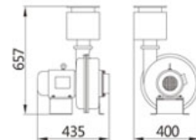
Blower B-200
