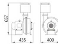
Blower B-200
