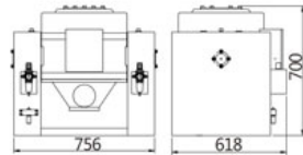
Shaker ET-3-230
