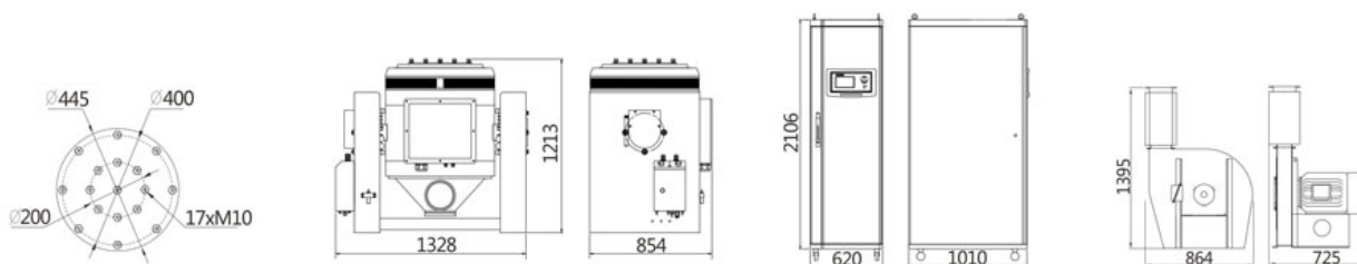
Shaker ET-30LS4-445
