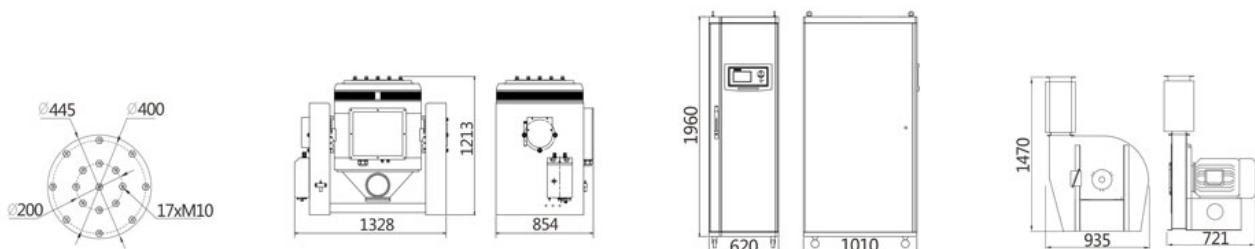
Shaker ET-40LS4-445
