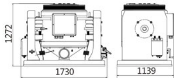
Shaker ET-50-445
