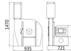
Blower B-5000
