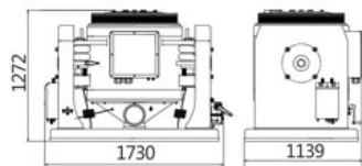
Shaker ET-60-445
