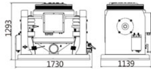
Shaker ET-60LS3-445
